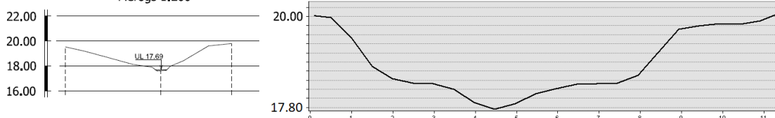
Grāvja (Ailes strauts) virsmas šķēršprofils Nr.1 (2.vieta)
