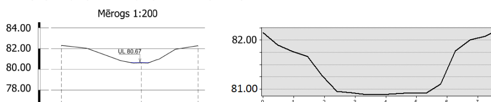
Grāvja (Mellupīte) virsmas šķērsprofils Nr. 2 (3.vieta)
