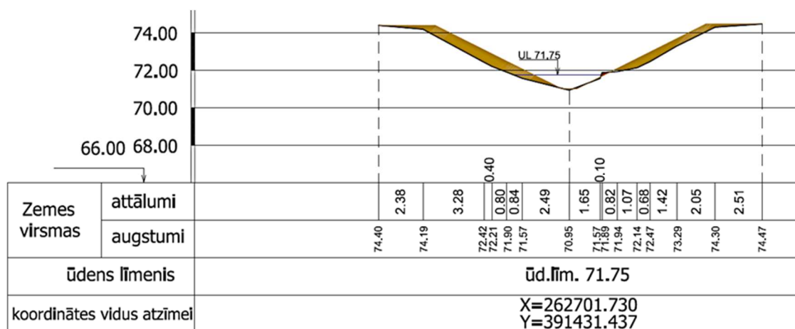
60.att. Grāvja (Mellupīte) virsmas šķērsprofils ar vēsturisko informāciju Nr.2 (1. vieta)
