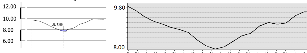
Grāvja (Bērze) virsmas šķēršprofils Nr. 1 (2.vieta)
