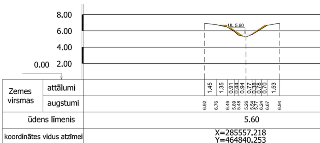
62.att. Grāvja (Bērze) virsmas šķērsprofils ar vēsturisko informāciju Nr.1 (3.vieta)
