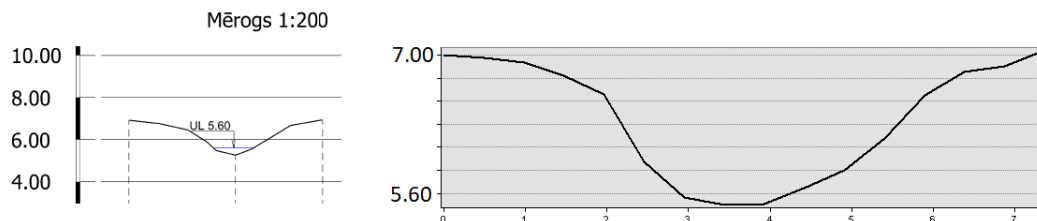
Grāvja (Bērze) virsmas šķērsprofils Nr. 1 (3.vieta)
