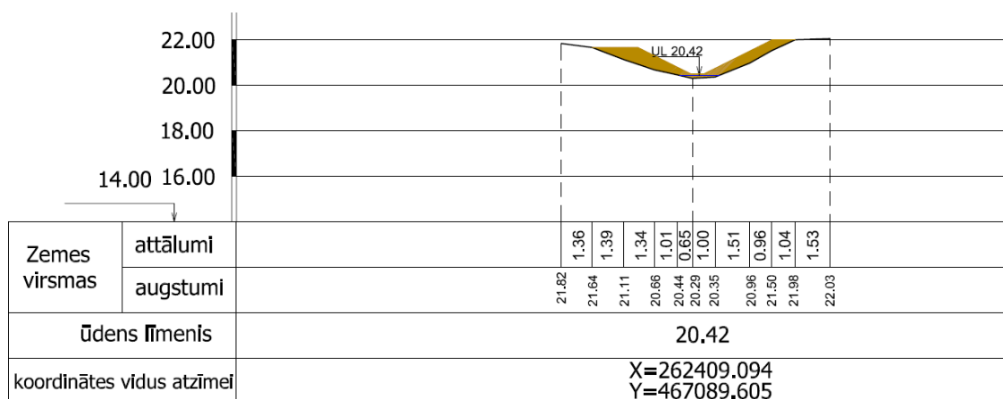
69.att. Grāvja (Ailes strauts) virsmas šķērsprofils ar vēsturisko informāciju Nr.2 (2. vieta)
