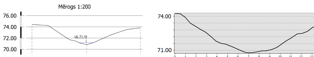
Grāvja (Mellupīte) virsmas šķērsprofils Nr. 1 (1.vieta)
