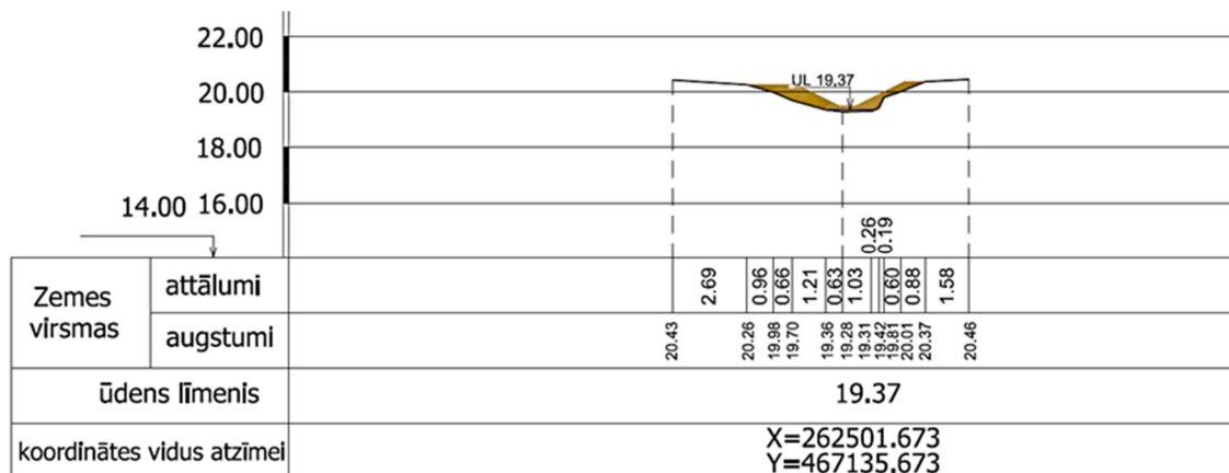
69.att. Grāvja (Ailes strauts) virsmas šķērsprofils ar vēsturisko informāciju Nr.2 (2. vieta)
