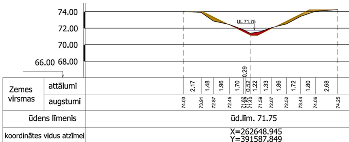
61.att. Grāvja (Mellupīte) virsmas šķērsprofils ar vēsturisko informāciju Nr.3 (1. vieta)
